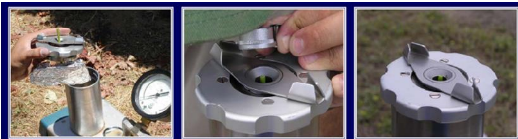
Figura II.4: Colocación de la hoja en la cámara de presión, (a) observación con lupa, y (b) determinación del potencial agua de la hoja a la presión en que se produce la aparición de una gota de agua en el corte del pecíolo de la hoja (c).
