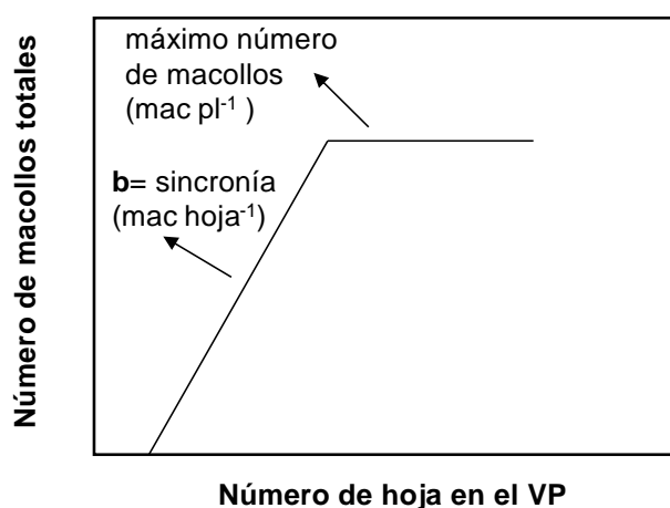
Figura 3.4. Esquema de la relación entre el número de macollos por planta y el número de hojas. Se detallan los principales parámetros cuantificados al realizar un ajuste utilizando Ec. 4.
