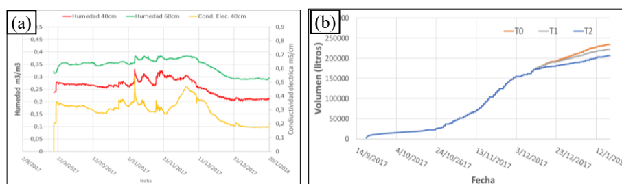
Fig. 7. Seguimiento de las aplicaciones de riego. (a) Evolución de variables en el suelo en el tratamiento testigo (T0); nivel de humedad a 40cm y 60cm de profundidad, y conductividad eléctrica a 40cm de profundidad. (b) Cantidad de agua aportada en cada tratamiento de riego
