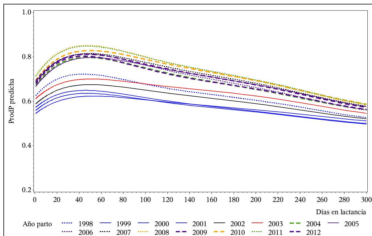
Figura 3.49. Producción de proteína predicha según modelo pol6 promedio según año de parto. ProdP: producción de proteína.
