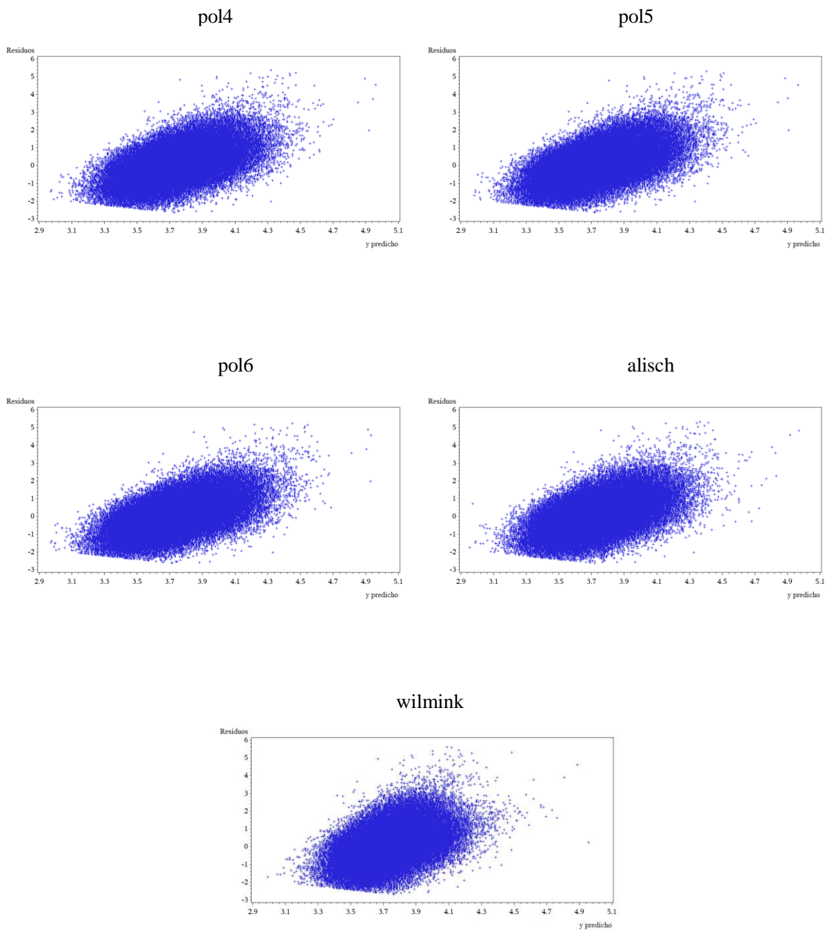
Figura 3.16. Residuos vs porcentaje de grasa predicha, para los modelos pol4, pol5 pol6, alisch y wilmink.
