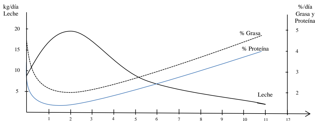
Figura 2.2. Curva de lactancia de las variables productivas producción de leche, porcentaje de grasa y proteína.
