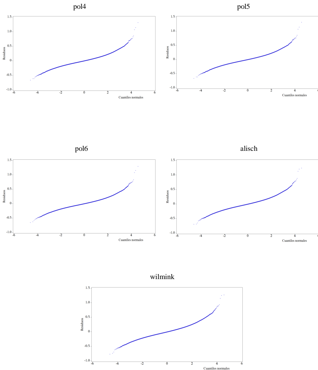
Figura 3.9. Gráfico de Probabilidad Normal del residuo de la variable producción de proteína, para los modelos pol4, pol5 pol6, alisch y wilmink.
