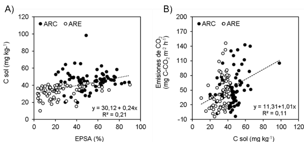
Figura 5. Regresión lineal entre los contenidos de carbono orgánico soluble (C sol) y A) el espacio poroso saturado con agua (EPSA) y B) las emisiones de \text{CO}_2 desde los suelos. Los símbolos llenos y vacíos corresponden a los suelos de textura arcillosa y arenosa, respectivamente. Las líneas punteadas representan la regresión entre variables. ARC: suelos arcillosos, ARE: suelos arenosos.
