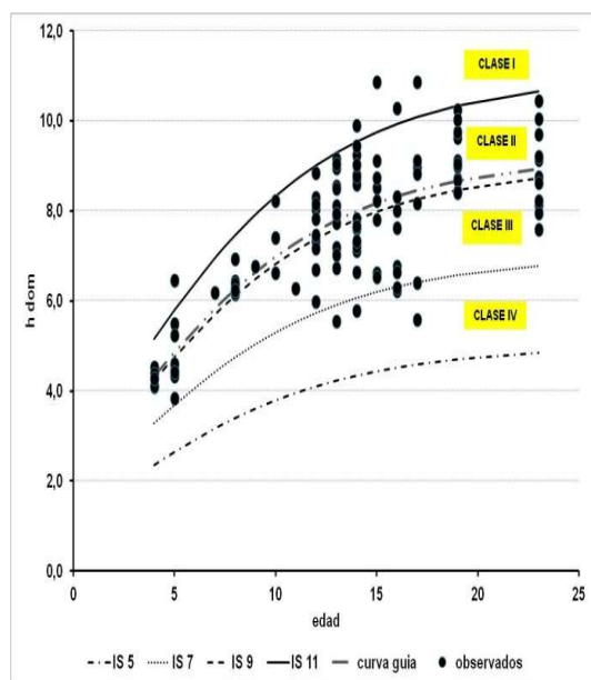
Gráfico 2. Curvas de índice de sitio. Graphic 2. Site index curves
