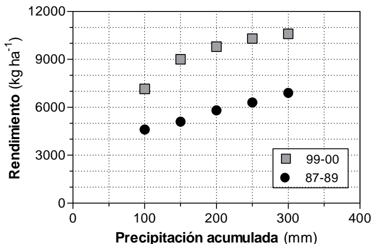
Figura 35: Relación entre el rendimiento de maíz y la disponibilidad de precipitaciones en un periodo de 50 días alrededor de la floración para establecimientos CREA del sur de la Provincia de Buenos Aires en las campañas 1987-1989 y 1999-2000. Los datos fueron obtenidos a partir de las ecuaciones presentadas en Calviño et al. (2003).
