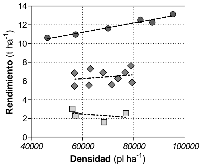
Figura 37: Rendimiento de maíz en función de la densidad de plantas para tres ambientes que difieren en el nivel de restricción hídrica alrededor de floración: i) restricción severa (línea inferior), restricción media y restricción leve (línea superior). Adaptado de Andrade et al. (1996).
