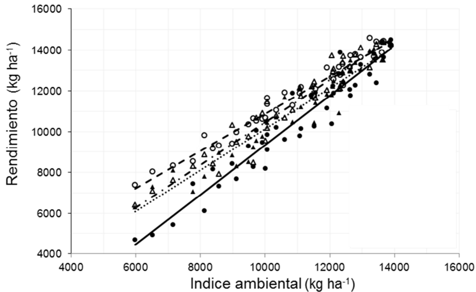
Figura 32. Rendimientos medios y ajustes lineales de 4 híbridos de maíz de estabilidad contrastante en función de un índice que refleja la productividad del ambiente (Castro, 2013).
