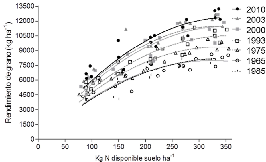
Figura 33: Relación entre rendimiento en grano y el nitrógeno disponible (incluye el del fertilizante, el presente en el suelo a la siembra y el mineralizado durante el ciclo del cultivo) para híbridos de distintas épocas sembrados con la densidad de selección y recomendación para alta producción (Ferreyra, 2015). Los años de liberación de los híbridos están indicados en la parte superior derecha del gráfico.
