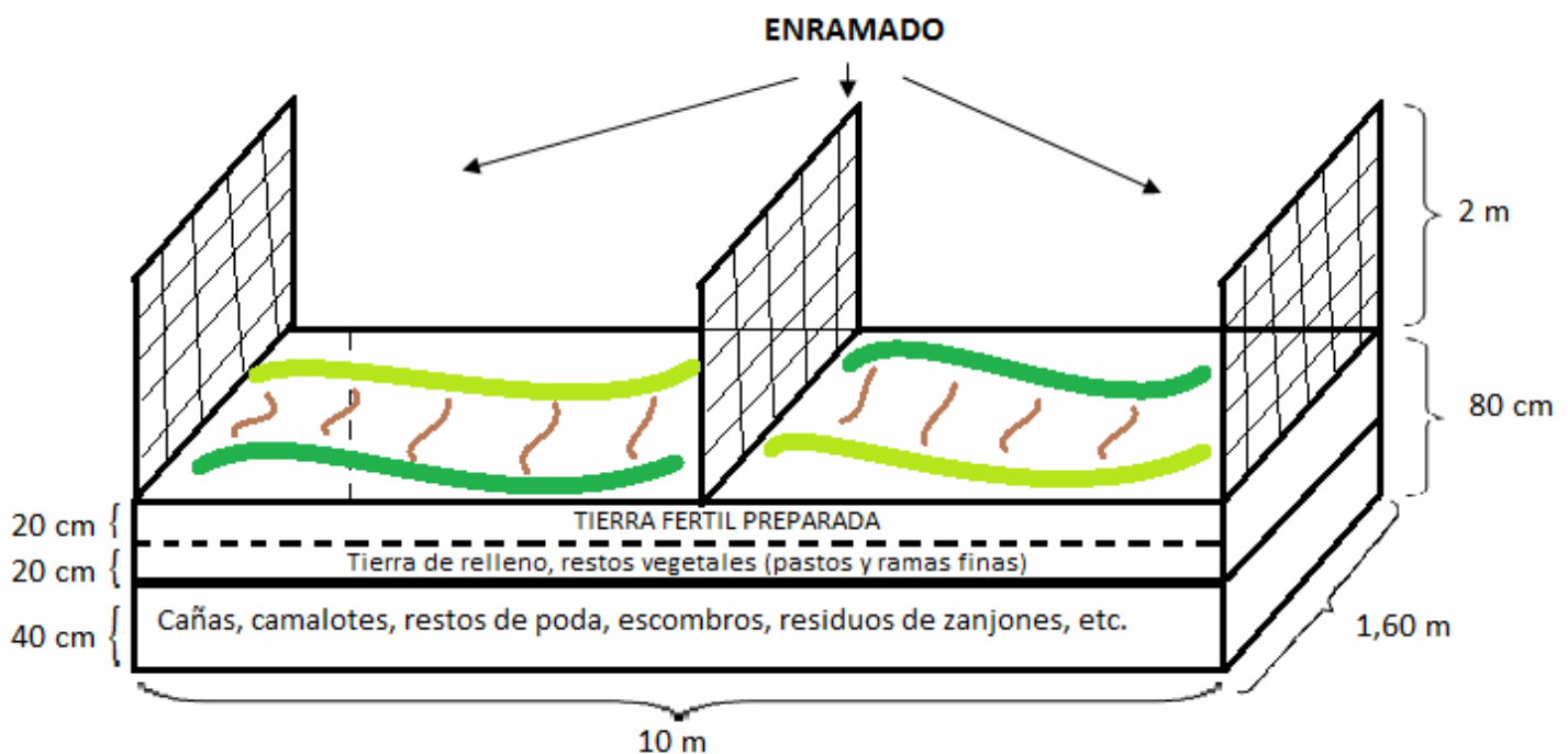
Figura 1: Esquema de huerta en altura
