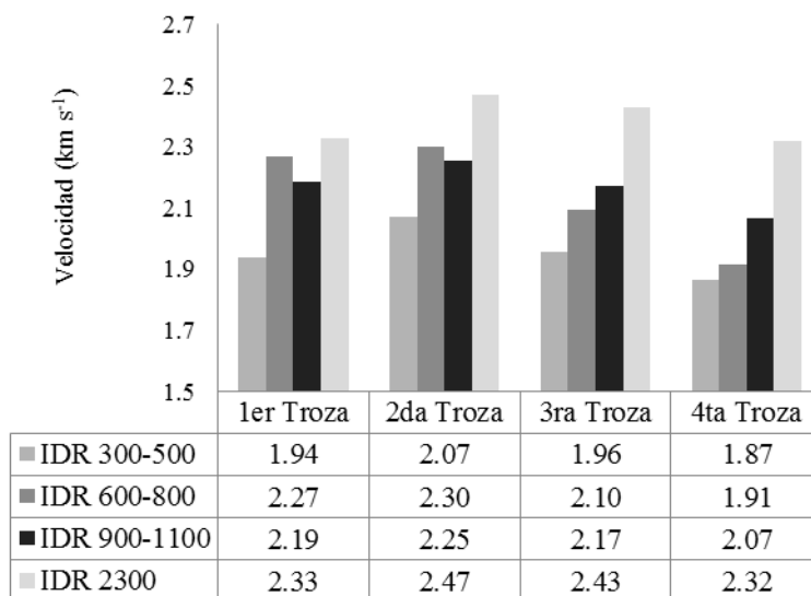
Figura 1. Velocidad de propagación de onda acústica (km s -1 ) en trozas de pino ponderosa según la densidad de manejo establecida en rango de Índice de Densidad de Rodal de Reineke (IDR). La primera troza corresponde a la base del árbol. IDR: 300-500; 600-800; 900-1100 y 2300 (Testigo). Ea. Sta. Lucía, Meliquina, Neuquén.
