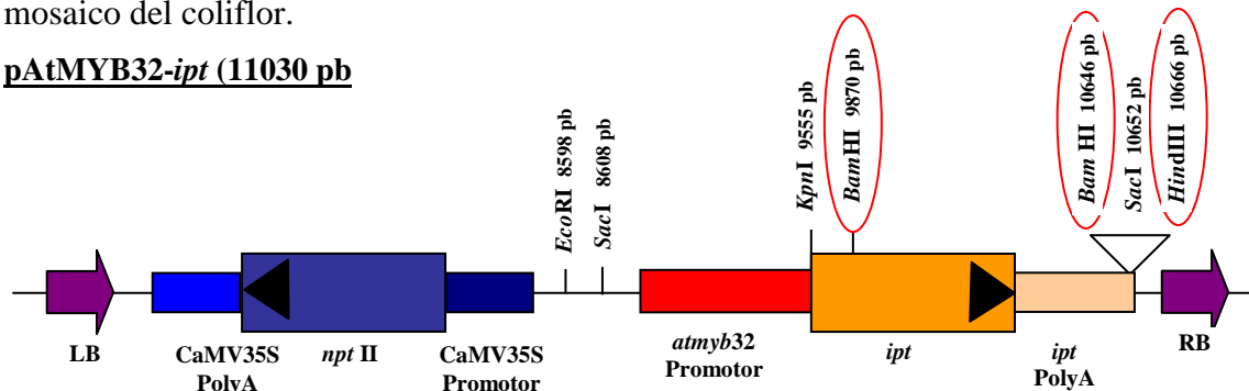
Figura 8- Mapa de restricción del T-DNA del vector binario pAtMYB32- ipt .
