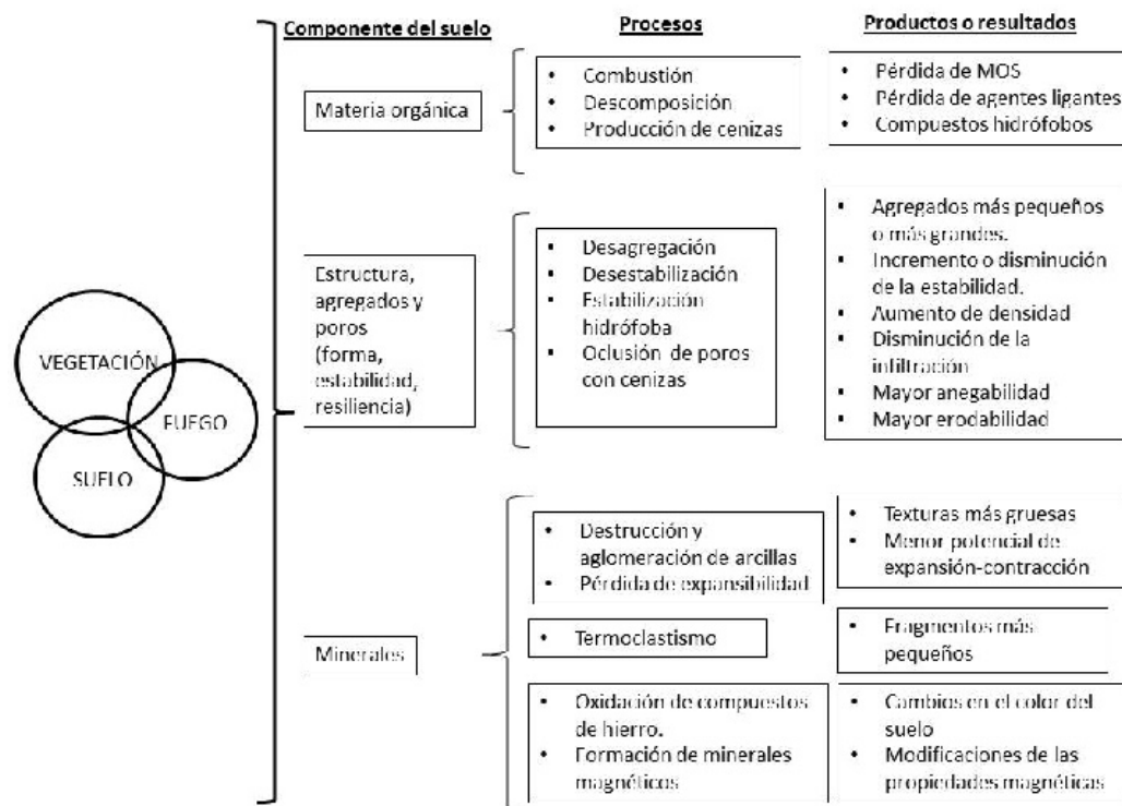
Figura 2. Esquema que resume los procesos que afectan a diversos componentes del suelo como consecuencia del fuego, y los productos o resultados que se derivan.
