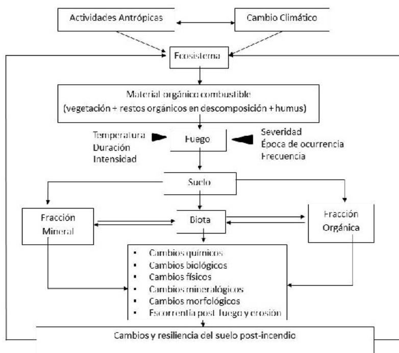
Figura 1. Esquema que resume los factores y los efectos del fuego generado por combustión de diferentes materiales orgánicos sobre los componentes y las propiedades del suelo.
