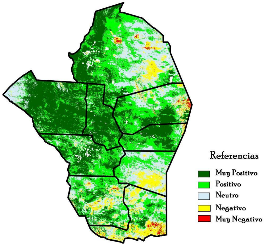
Figura 2.2. Anomalías de NDVI segunda quincena Noviembre 2019.
