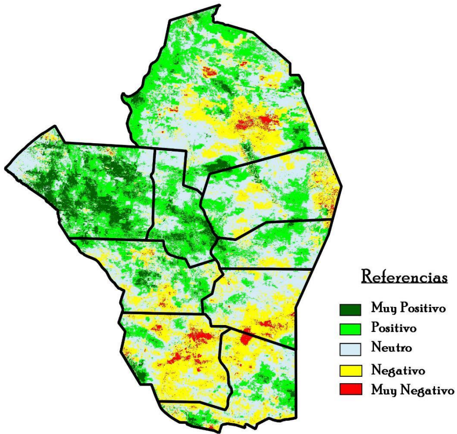
Figura 2.4. Anomalías de NDVI segunda quincena Diciembre 2019.
