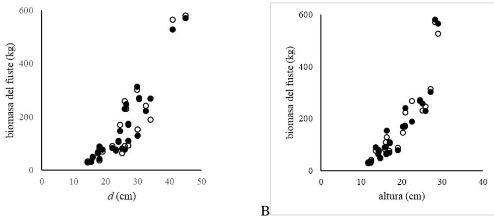
Figura 3. A.- Valores observados (○) y estimados (●) de biomasa del fuste en función del diámetro a la altura de pecho ( d ). B.- Valores observados (○) y estimados (●) de biomasa del fuste en función de la altura
