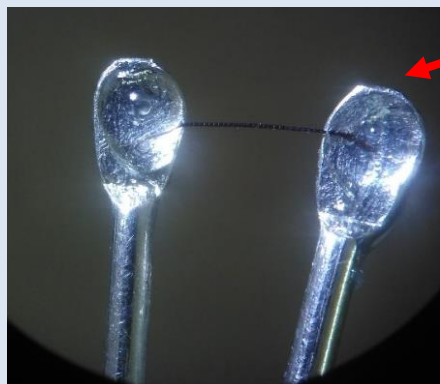
Electro-anteno-detector
