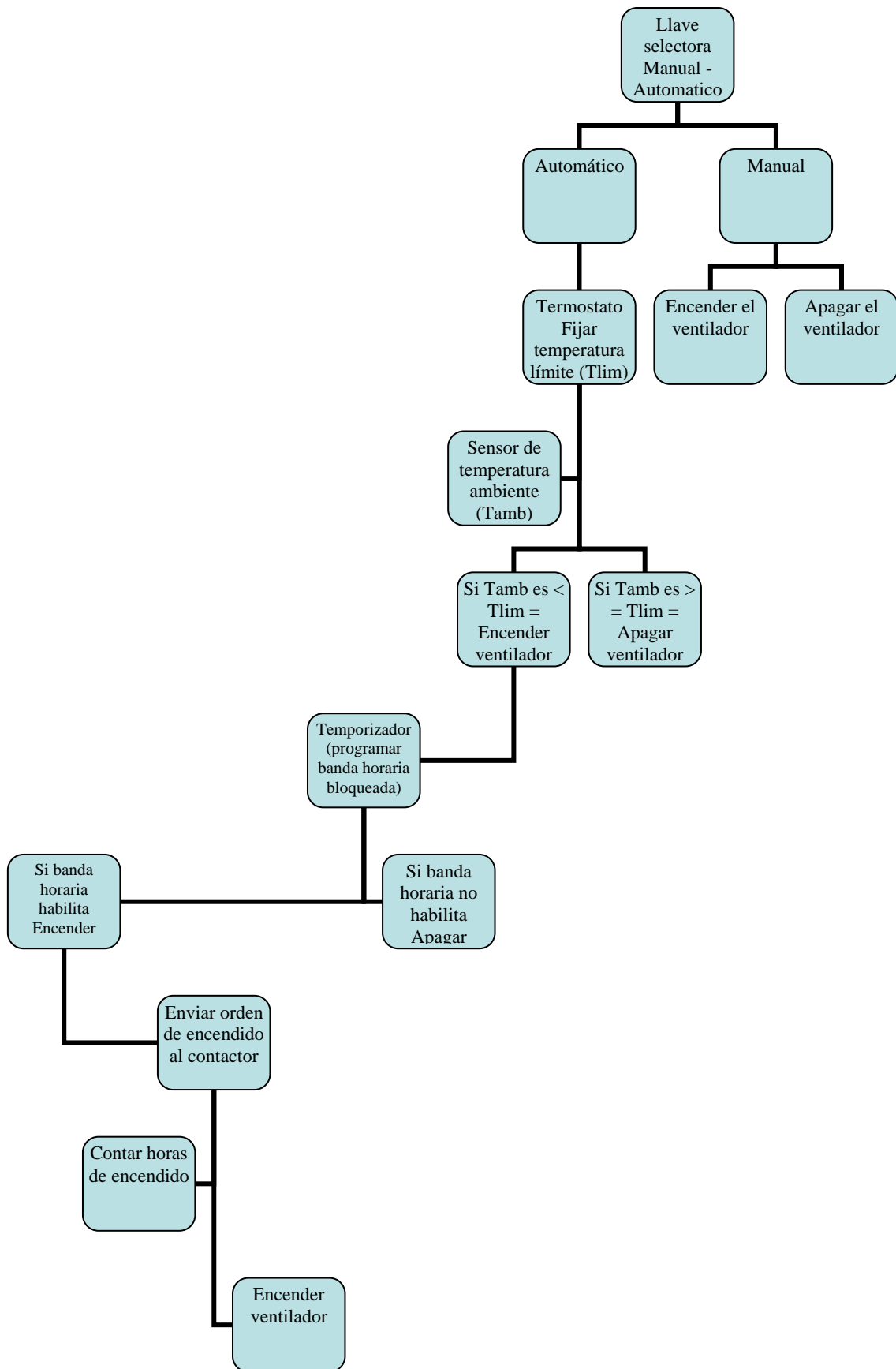
Figura 2. Diagrama de secuencia de decisiones del controlador automático de aireación.
