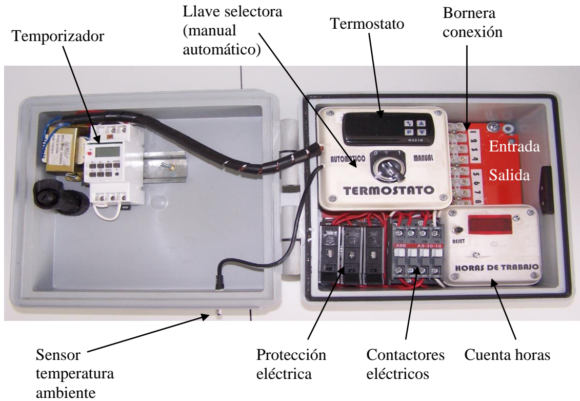
Figura 3. Controlador de aireación con el detalle de sus componentes.
