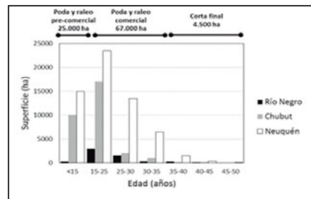
Figura 2. Distribución en clases de edad de las forestaciones con pino ponderosa establecidas en Neuquén, Río Negro y Chubut (actualizado a 2019 a partir de Loguercio y Deccechis 2006).
