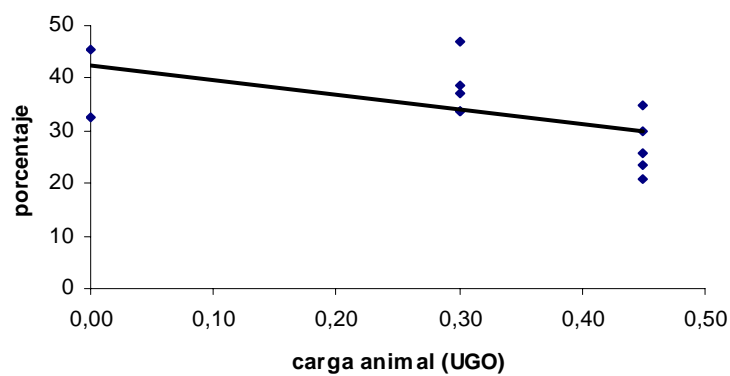
Figuras N° 3-7 efecto de la carga animal sobre los índices de función del paisaje. (A) Estabilidad ( R^2= 0.164 p= 0.191 ); (B) Infiltración ( R^2= 0.349 p= 0.0429 ); (C) Reciclaje ( R^2= 0.327 p=0.0519 ).
