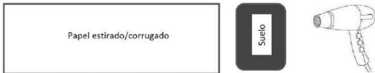
Figura 2.05. Esquema de dispositivo casero para evaluar el efecto del tamaño de partícula y humedad del suelo sobre la susceptibilidad a la erosión eólica.
