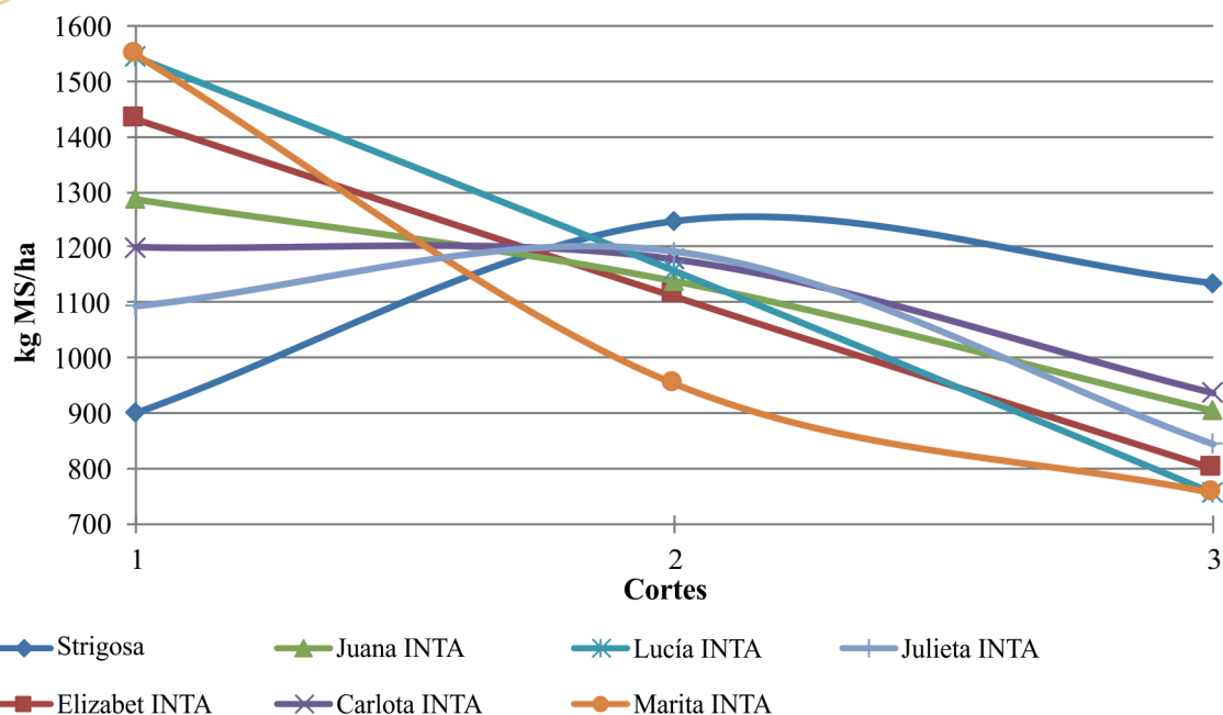
Figura 1. Curva de producción de MS de avenas con tres cortes.
