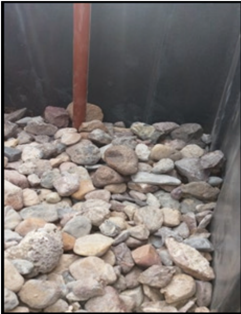
. Materiales utilizados como filtros; a las izquierda la grava y a la derecha el relleno para biodigestores tipo biolam
