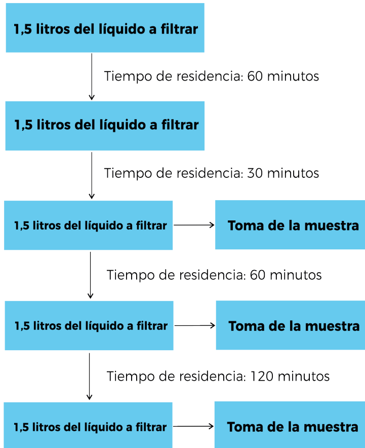
. Esquema del ensayo de filtrado número 2
