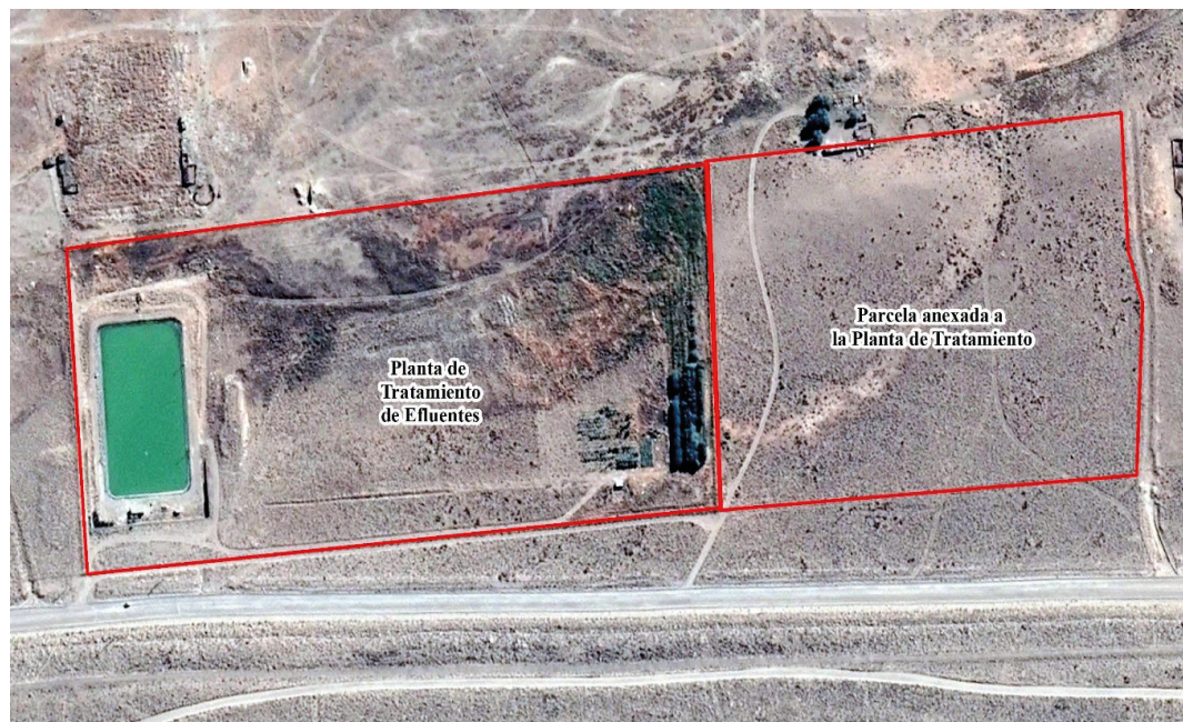
. Planta de tratamiento y parcela anexada para reuso de efluente en riego
