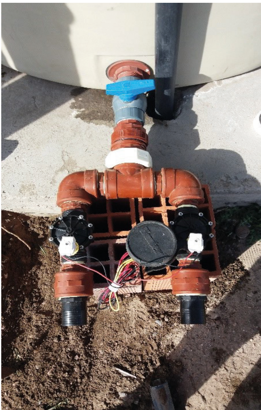
. Automatización con Programador, electroválvulas y solenoides para baja presión
