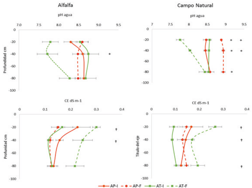
. Variación del pH y la CE del suelo en alfalfa y campo natural, regados con agua tratada (AT) y Agua de perforación (AP) al inicio (I) y luego de tres temporadas de riego (F)
