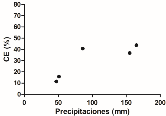
Figura 2.9. Coeficientes de escurrimiento (CE) (%) para los eventos evaluados en el periodo analizado (junio de 2016 a diciembre de 2017).
