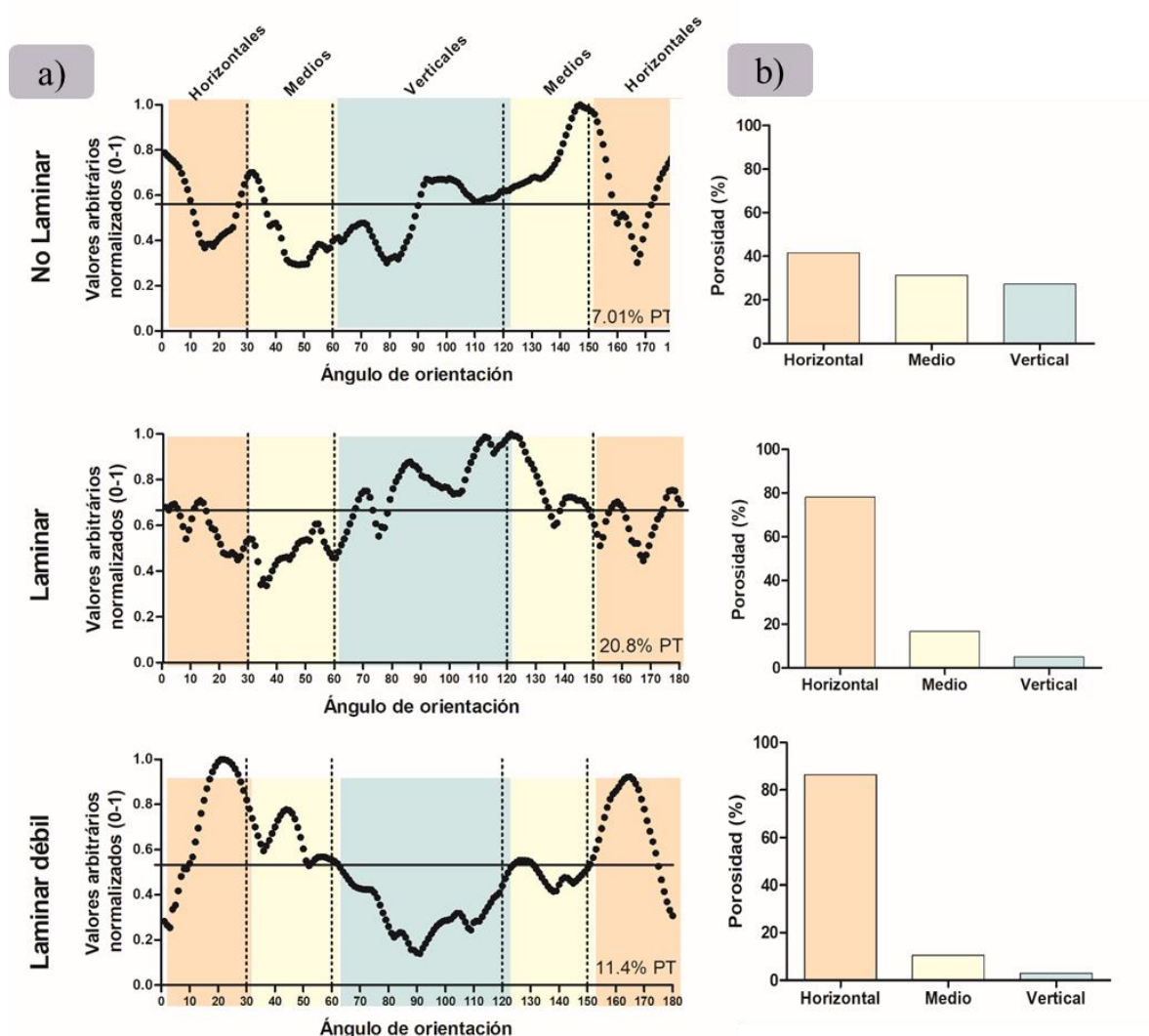
Figura 3.20. Orientación de los poros elongados mediante a) el programa JMicro Vision v1.2 y b) el método RIMPAS (con ajustes Kraemer et al. , 2016) de las estructuras laminares débiles (LD), laminares (L) y no laminares (NL).
