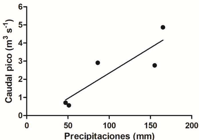
Figura 2.11. Relación entre las precipitaciones que provocaron escurrimientos y el caudal pico para el periodo analizado (junio de 2016 a diciembre de 2017).
