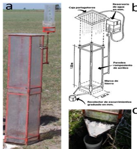
Figura 2.4. a) Simulador de lluvia; b) Esquema del equipo; c) Vista de la parcela y del recipiente recolector del escurrimiento.
