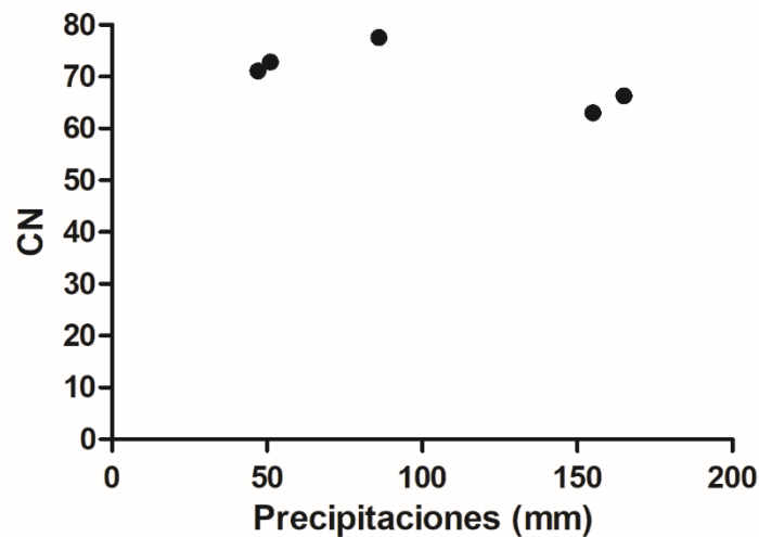
Figura 2.12. Valores de Número de curva (CN) para la microcuenca empleando el método de Hawkins (1993) para el periodo analizado (junio de 2016 a diciembre de 2017).
