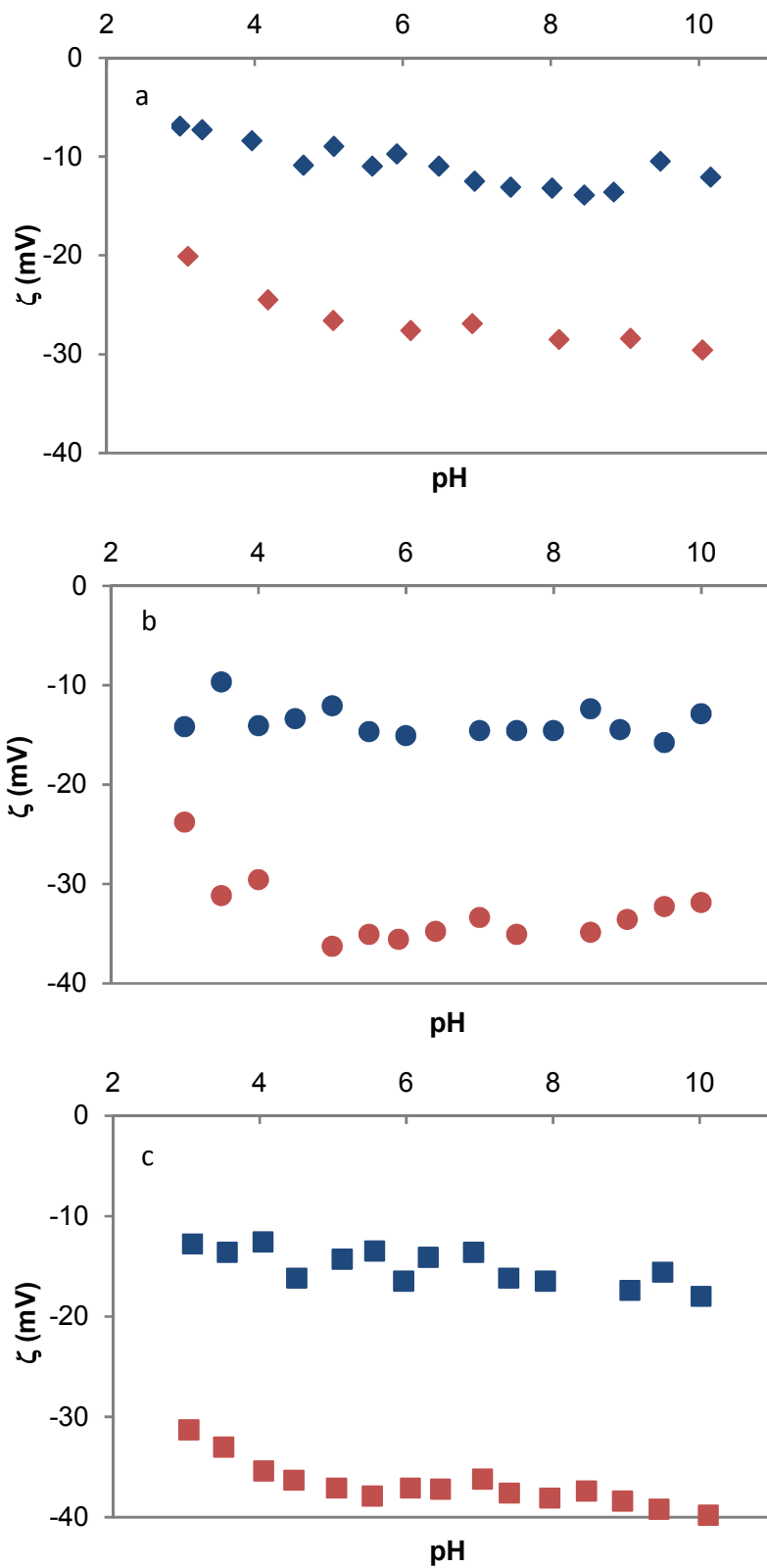
Figura 5.1. Potencial zeta de la fracción arcilla (a), del AH (a), y de la fracción arcilla más AH (c), en presencia de NaCl (series de color rojo) y \text{CaCl}_2 (series de color azul). (FI=0,01)
