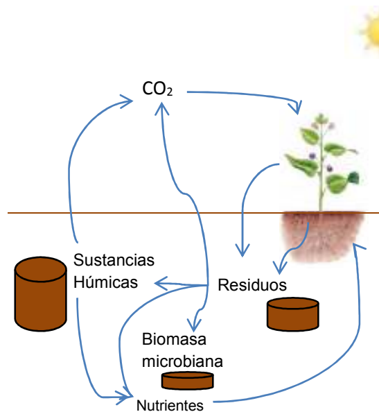
Figura 1.2. Principales flujos de carbono en el sistema suelo-planta-atmósfera.
