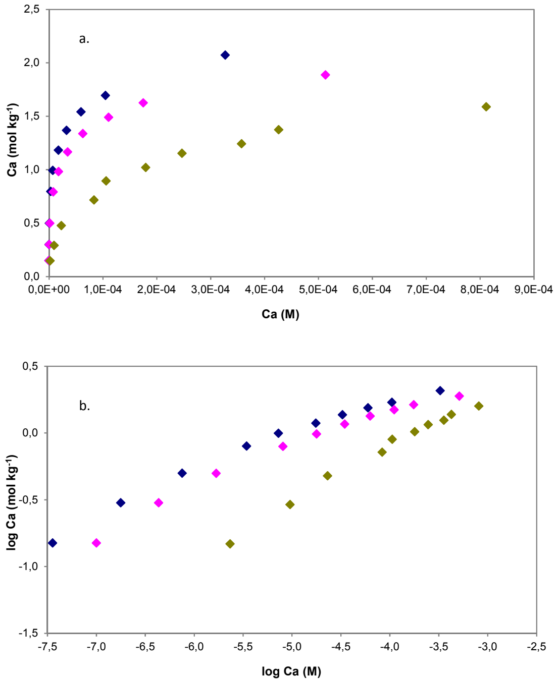
Figura 2.9. a) Isothermas de adsorción de calcio a AH a pH 5 (◆), 7 (◆) y 9 (◆). b) Representación logarítmica de las isothermas de adsorción mostradas en la Figura a).
