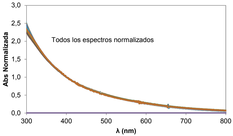
Figura 5A.4. Todos los espectros normalizados indicados en las Figuras 5A.1, 5A.2 y 5A.3. Los puntos por debajo de \lambda 390 nm correspondientes a los cuatro espectros normalizados que presentan ruido en la señal de la Figura 5A.3 no se muestran en esta figura para mayor claridad.
