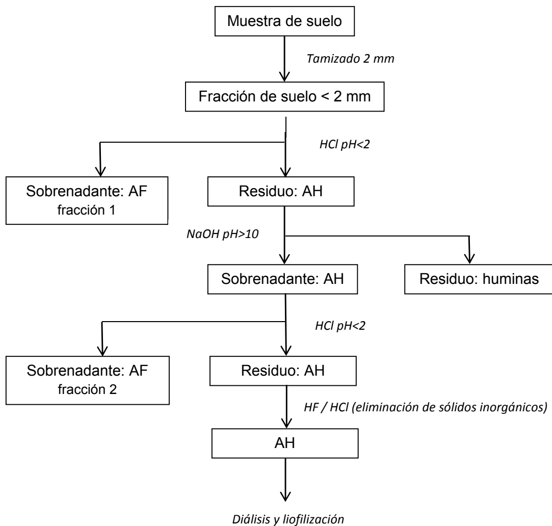
Figura 2.2. Esquema general de las etapas del procedimiento de extracción y purificación del AH.
