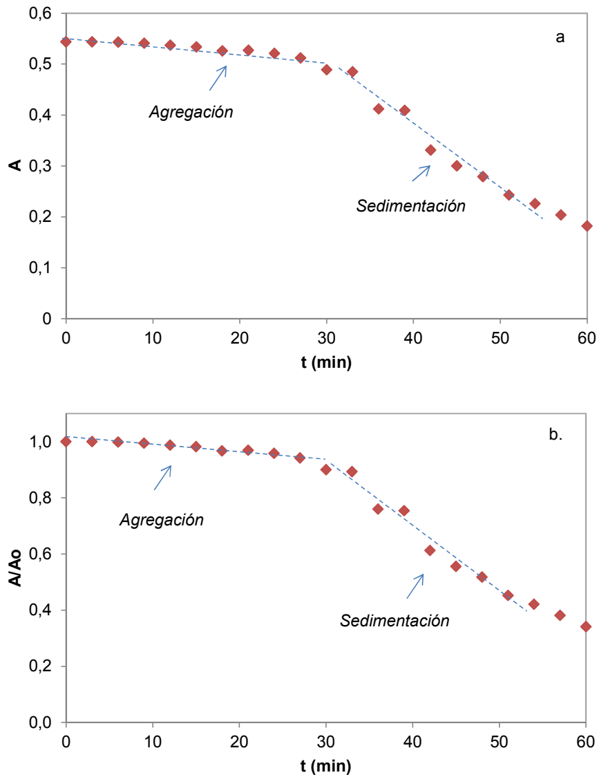
Figura 6.2. a) Absorbancia vs. tiempo de una suspensión de fracción arcilla 400 \text{ mg L}^{-1} en NaCl 0,4 \text{ M} a pH 7, b) absorbancia normalizada de fracción arcilla ( A/A_0 ) vs. tiempo para las condiciones experimentales indicadas en a). Las dos rectas que se dibujan representan las pendientes que corresponden a la fase de agregación y a la de sedimentación. El punto de cruce de las curvas, alrededor de 30 min, puede tomarse como el tiempo necesario para que los agregados que se forman sean lo suficientemente grandes como para comenzar a sedimentar.
