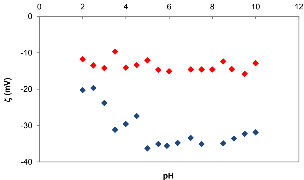
Figura 2.7. Efecto del pH sobre el potencial zeta del AH en NaCl (♦) y en CaCl 2 (♦) (FI=0,01).
