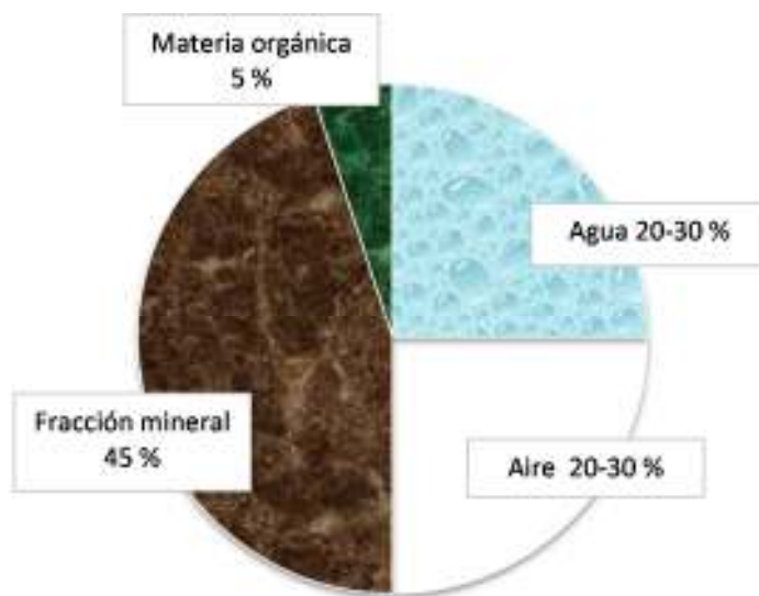
Figura 1.1. Fases del sistema suelo.
