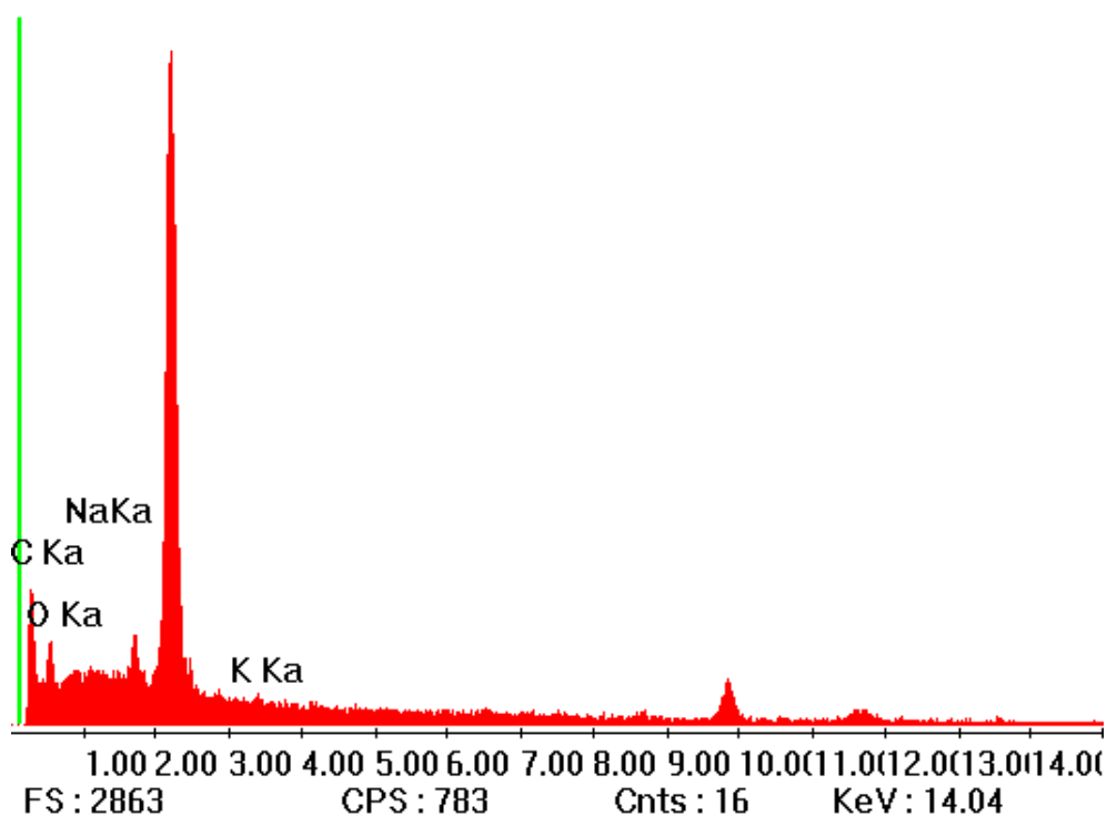
Figura 2.4. Espectro EDAX de partículas de AH, observadas en la Figura 2.3c.
