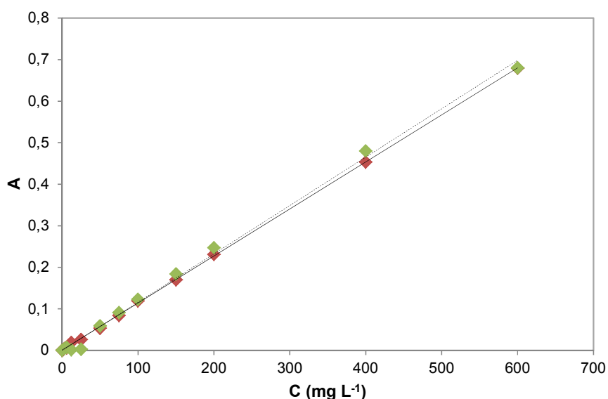
Figura 6.1. Curvas de calibración Absorbancia vs. concentración de fracción arcilla obtenidas con un espectrofotómetro Metrolab 1600 (♦) y Perkin Elmer Lambda35 (◆).
