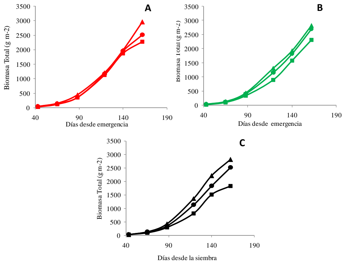
Figura 3: Producción de biomasa durante el ciclo del cultivo para el tratamiento con DLR 0.8 (A), DLR 1.05 (B) y DLR 1.6 m (C). Los triángulos, círculos y cuadrados indican la producción de biomasa total para el primer, segundo y tercer tercio.
