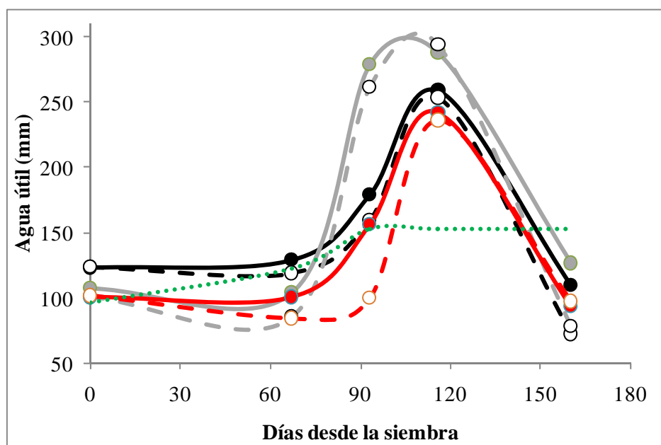
Figura 2. Agua útil obtenida en el perfil de suelo explorado por las raíces del cultivo durante el ciclo. Las líneas negras representan al tratamiento de DLR 0.8, las grises a DLR 1.05 y las rojas a DLR 1.6. Las líneas Llenas indican el contenido de agua al lado del lateral de riego, y las entrecortadas en la entrelínea. La línea verde punteada indica el umbral de riego que representa el 50% del agua útil.
