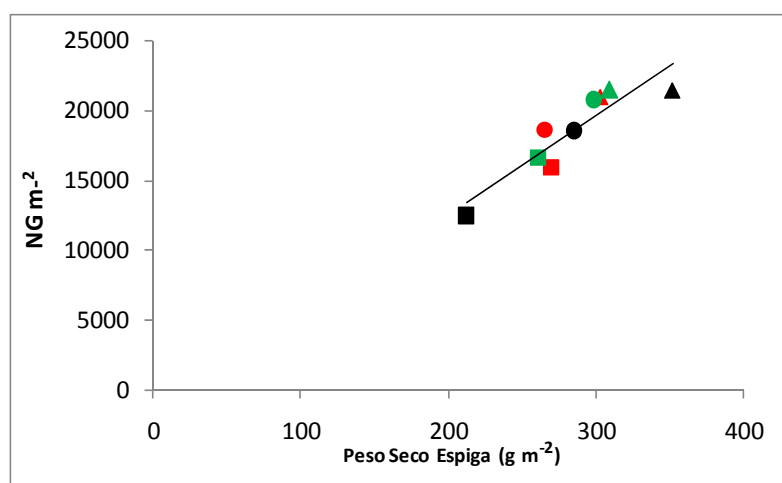
Figura 4. Relación entre el peso seco de la espiga al final del período crítico y el número de granos por metro cuadrado. Los símbolos rojos representan al tratamiento de DLR 0,8 m, los verdes a DLR 1,05 y los negros a DLR de 1.6m. Los círculos representan el primer tercio, los triángulos al segundo tercio y los cuadrados al tercer tercio.
