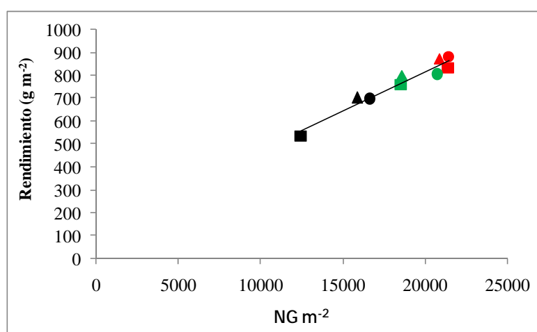
Figura 5. Relación entre el número de granos por metro cuadrado y el rendimiento del cultivo. Los símbolos rojos representan al tratamiento de DLR 0,8 m, los verdes a DLR 1,05 y los negros a DLR de 1,6m. Los círculos representan el primer tercio, los triángulos al segundo tercio y los cuadrados al tercer tercio.
