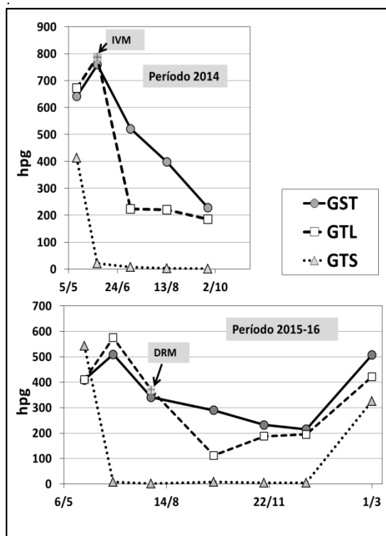
Figura 2. Media de los conteos de huevos (hpg) de la recría durante los periodos 2014 y 2015-16. GTS (Tratamiento sistémico), GTL (tratamiento local) y GST (sin tratamiento). IVM: tratamiento con ivermectina; DRM: tratamiento con doramectina.
