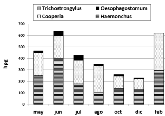
Figura 3. Promedio de la proporción de los géneros de nematodos recuperados de los coprocultivos según el hpg promedio durante todo el estudio.
