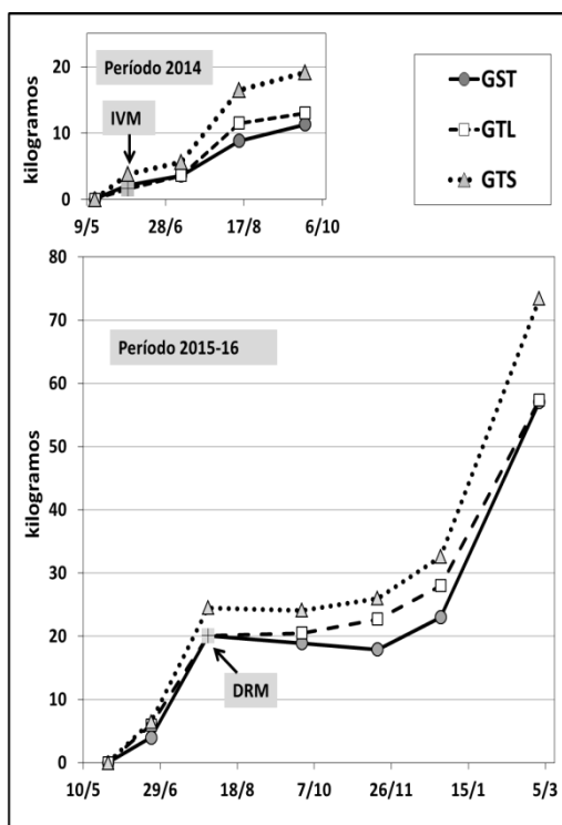
Figura 4. Ganancias de peso vivo en kg de las terneras en los períodos 2014 y 2015-16. GST: grupo sin tratamiento; GTS grupo con tratamiento sistemático con moxidectina; GTL grupo con el tratamiento del establecimiento.+ IVM: tratamiento con ivermectina; + DRM: tratamiento con doramectina.
