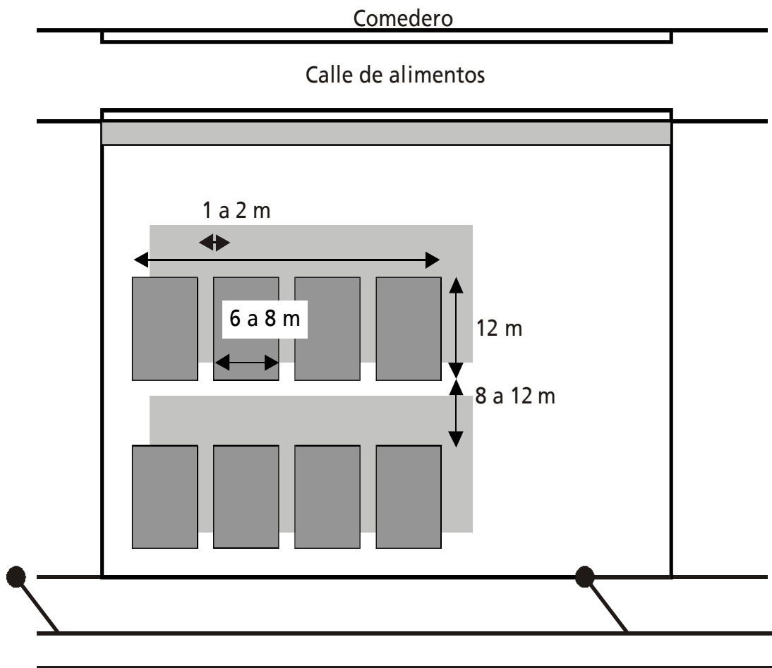
Tamaños sugeridos y ubicación de sombras artificiales
