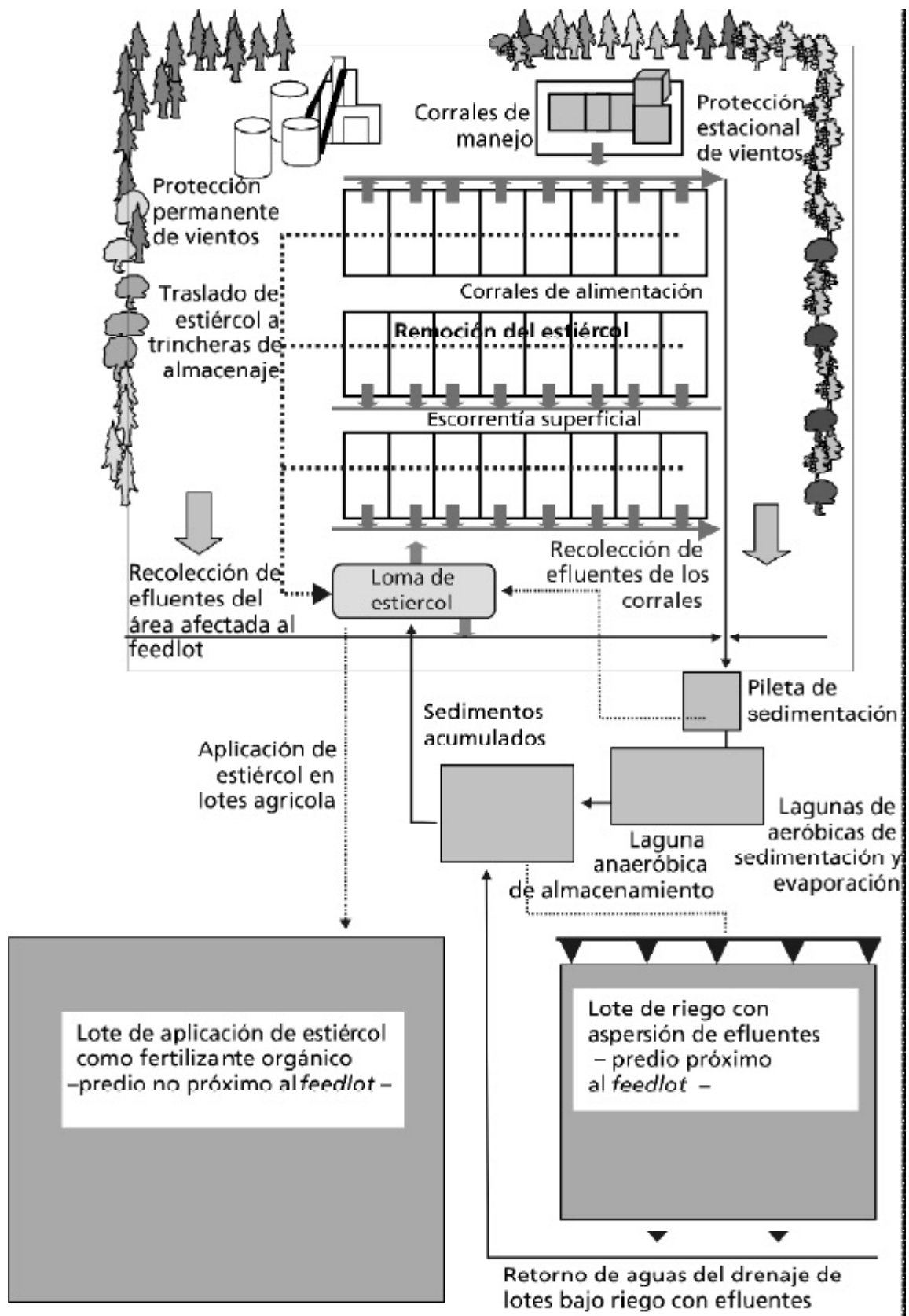
Figura 3.1. Esquema de una estructura de manejo de efluentes líquidos y de estiércol en el diseño de un feedlot
