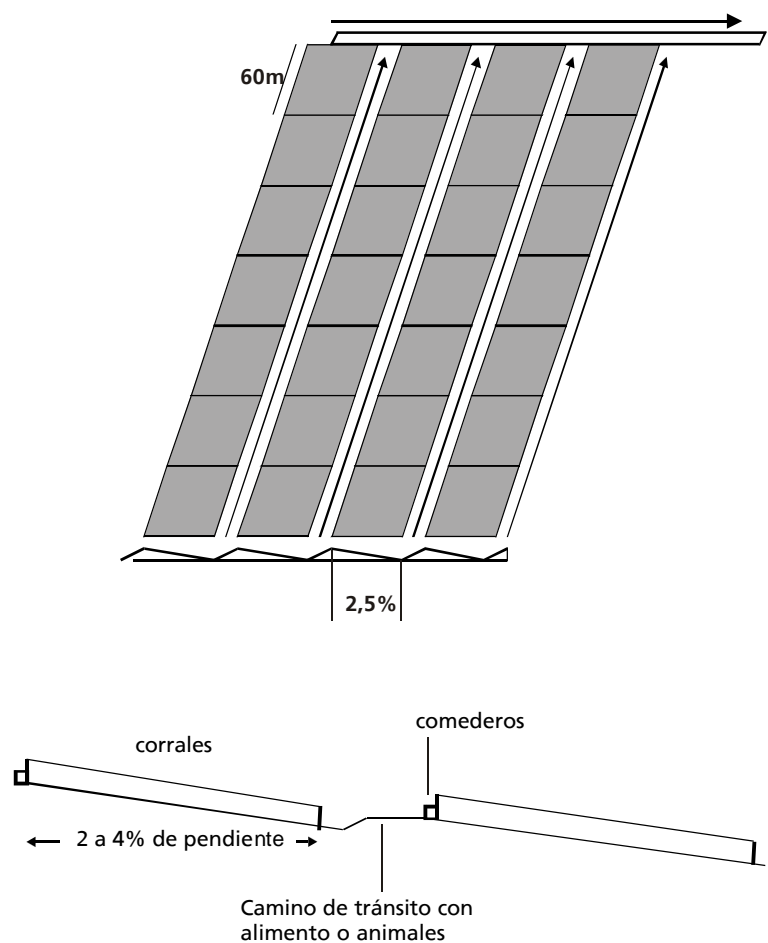
Diseño y ubicación espacial de los corrales
