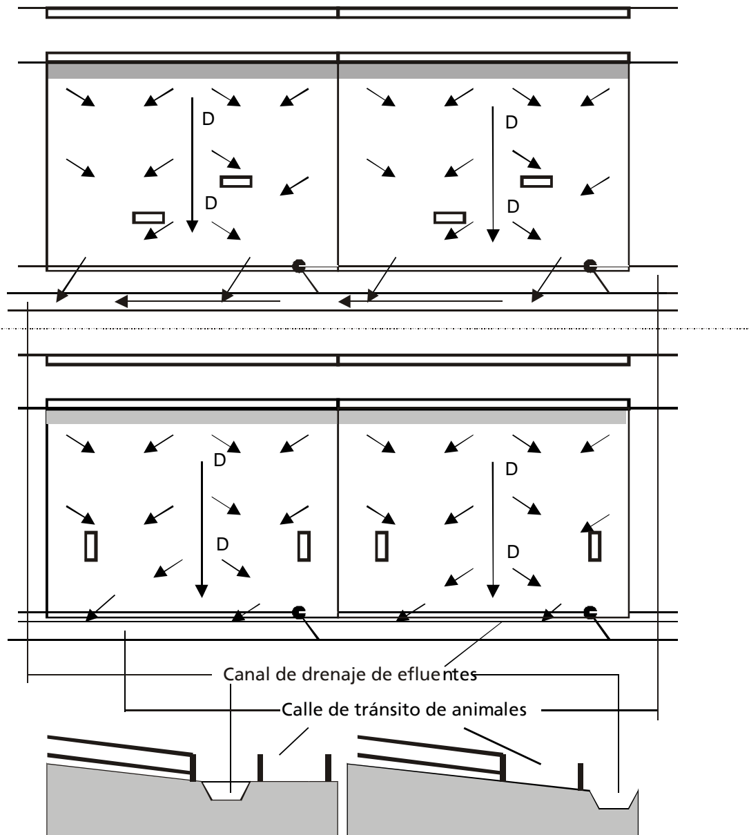
Diagrama del diseño del flujo de efluentes en escurrimiento superficial
