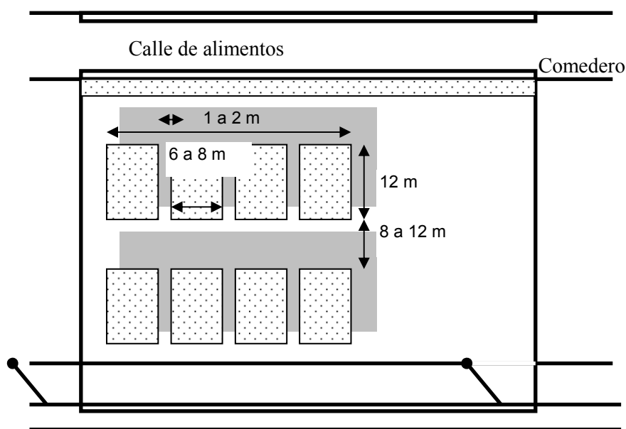
Tamaños sugeridos y ubicación de sombras artificiales
