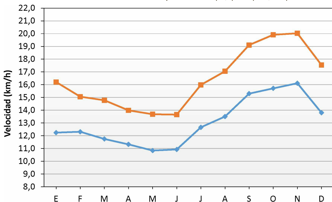
Figura N°4 Velocidad media mensual del viento a 2 y 10 m de altura (km/h). SMN (1961/2018)
