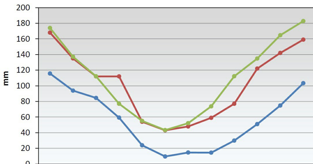
Figura N°17 Balance Hidrológico Mensual de Villa Mercedes. INTA EMC (1969/2012)
