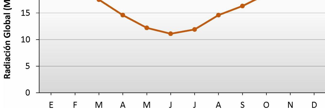
Cuadro N°12 Radiación global media mensual y anual (MJ/m 2 ). SMN (1958/2018)
