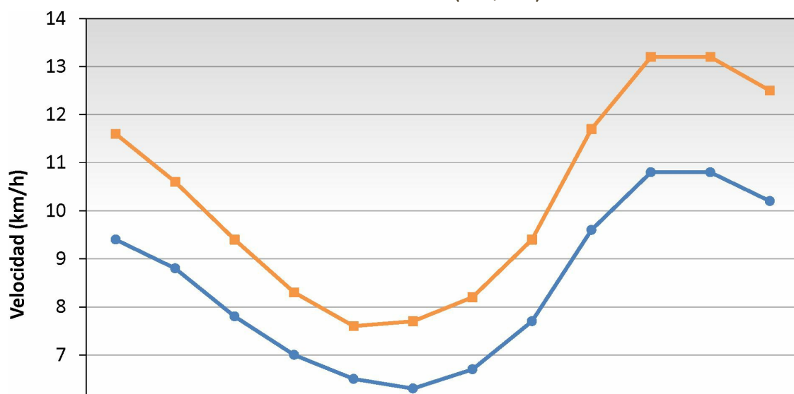
Figura N°5 Velocidad media mensual del viento a 2 y 10 m de altura (km/h) de Villa Mercedes INTA Villa Mercedes - EMC (1969/2013)
