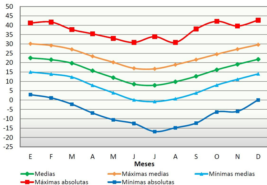
Figura N°9 Temperatura media, máxima y mínima media mensual y absolutas de Villa Mercedes (°C) INTA Villa Mercedes - EMC (1969/2013)
