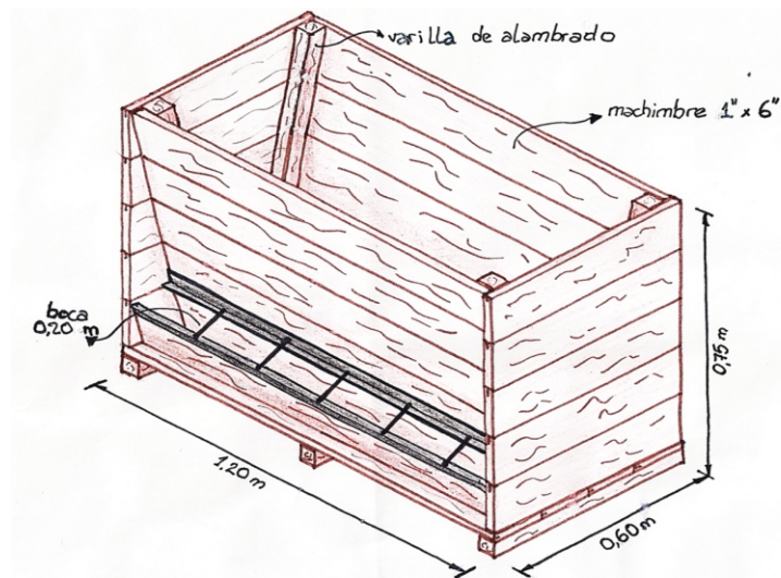
Croquis tolva para cachorros, 12 bocas, capacidad 200 kg
